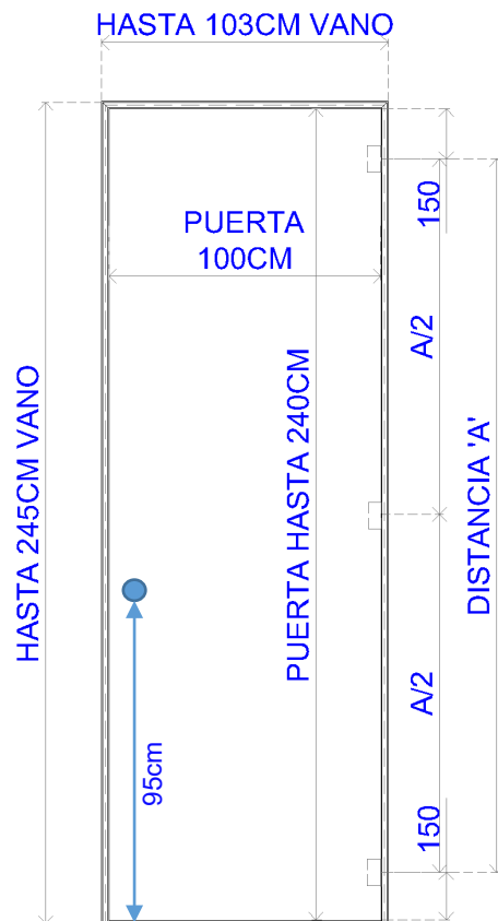
PUERTA SENCILLA
